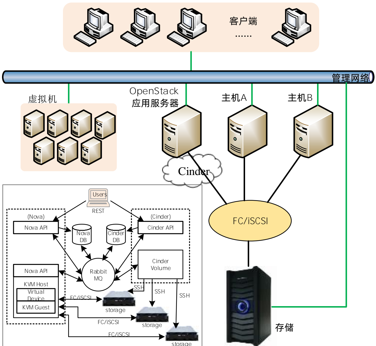
图 1-1 Cinder 主机插件应用拓扑图
